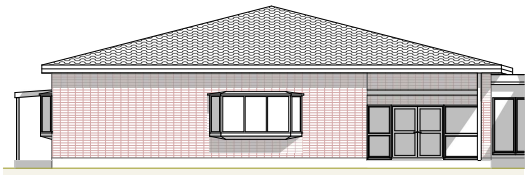
JULKISIVU LÄNTEEN 1:150
