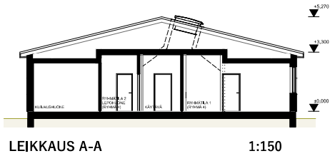
LEIKKAUS A-A
