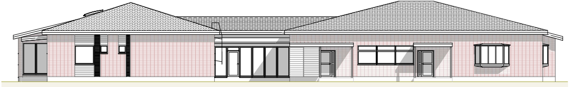
JULKISIVU POHJOISEEN 1:150
