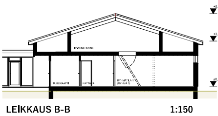
LEIKKAUS B-B
